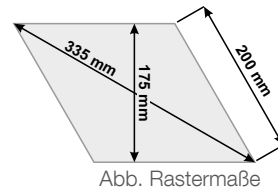
Abb. Rastermaße
